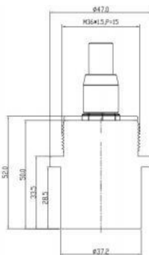
图 2-4 尺寸图 (不锈钢)
