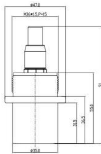
图 2-2 尺寸图
